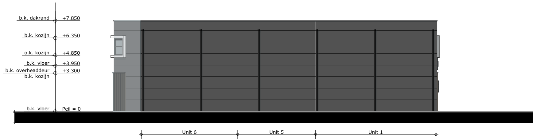
NOORD-WESTGEVEL
