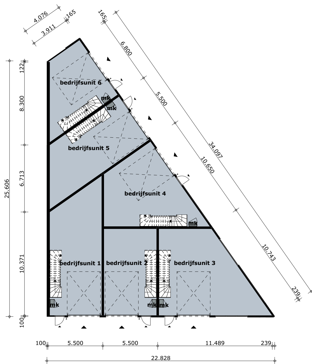
BEGANE GROND
