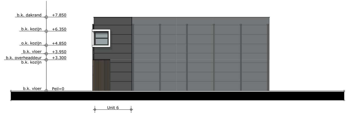
NOORDGEVEL
