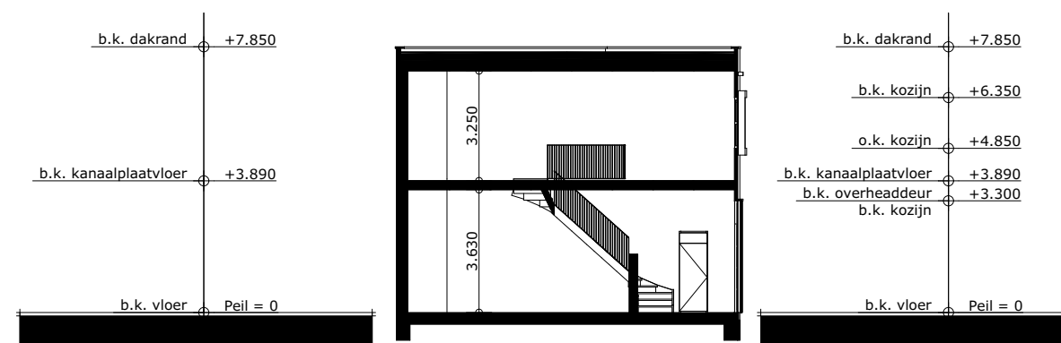
DOORSNEDE B-B
