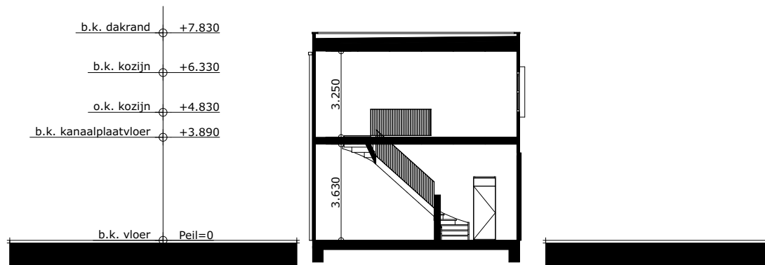
DOORSNEDE B-B
