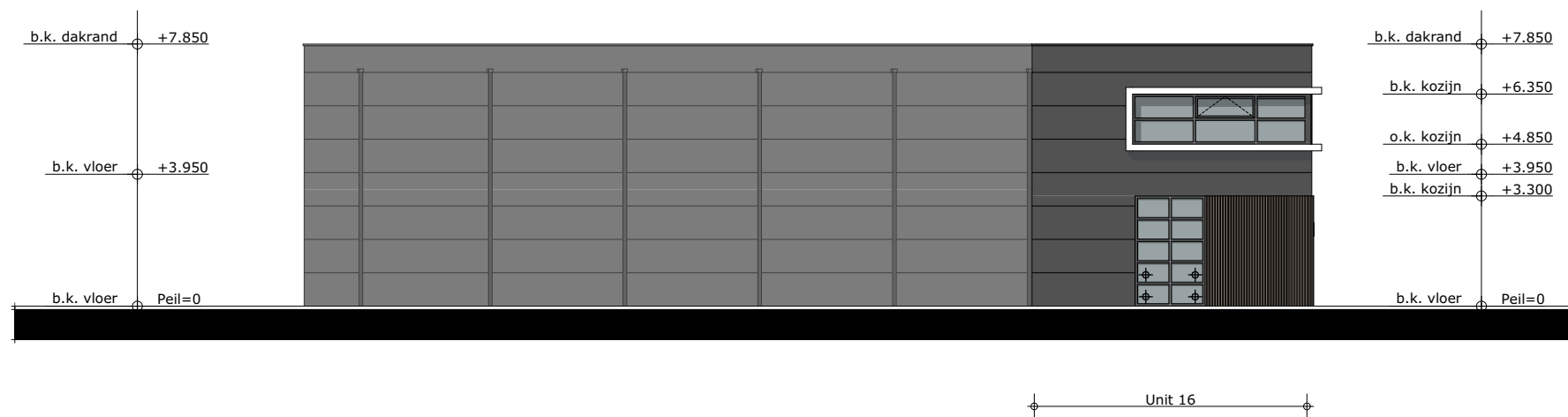
NOORD-OOSTGEVEL
